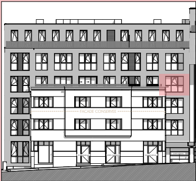
ELEVATION Avant
